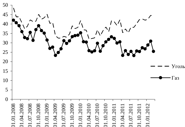
Рис. 8. Выработка электроэнергии по видам генерации в 16 странах Европы 8 , млрд кВт·ч в месяц
